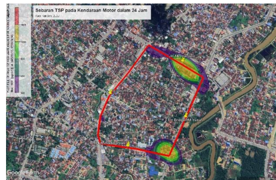
(b) Simulasi selama 24 jam
