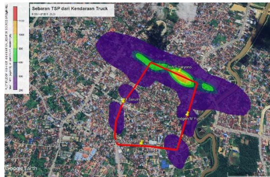
(a) Simulasi selama 1 jam
